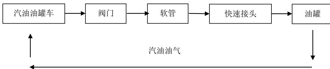
图 2.4.1-1 乙醇汽油罐车密闭卸油及卸油油气回收工艺流程图
