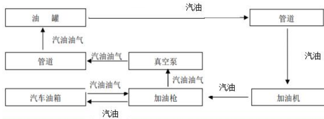
图 2.4.1-2 乙醇汽油加油及油气回收工艺流程图
