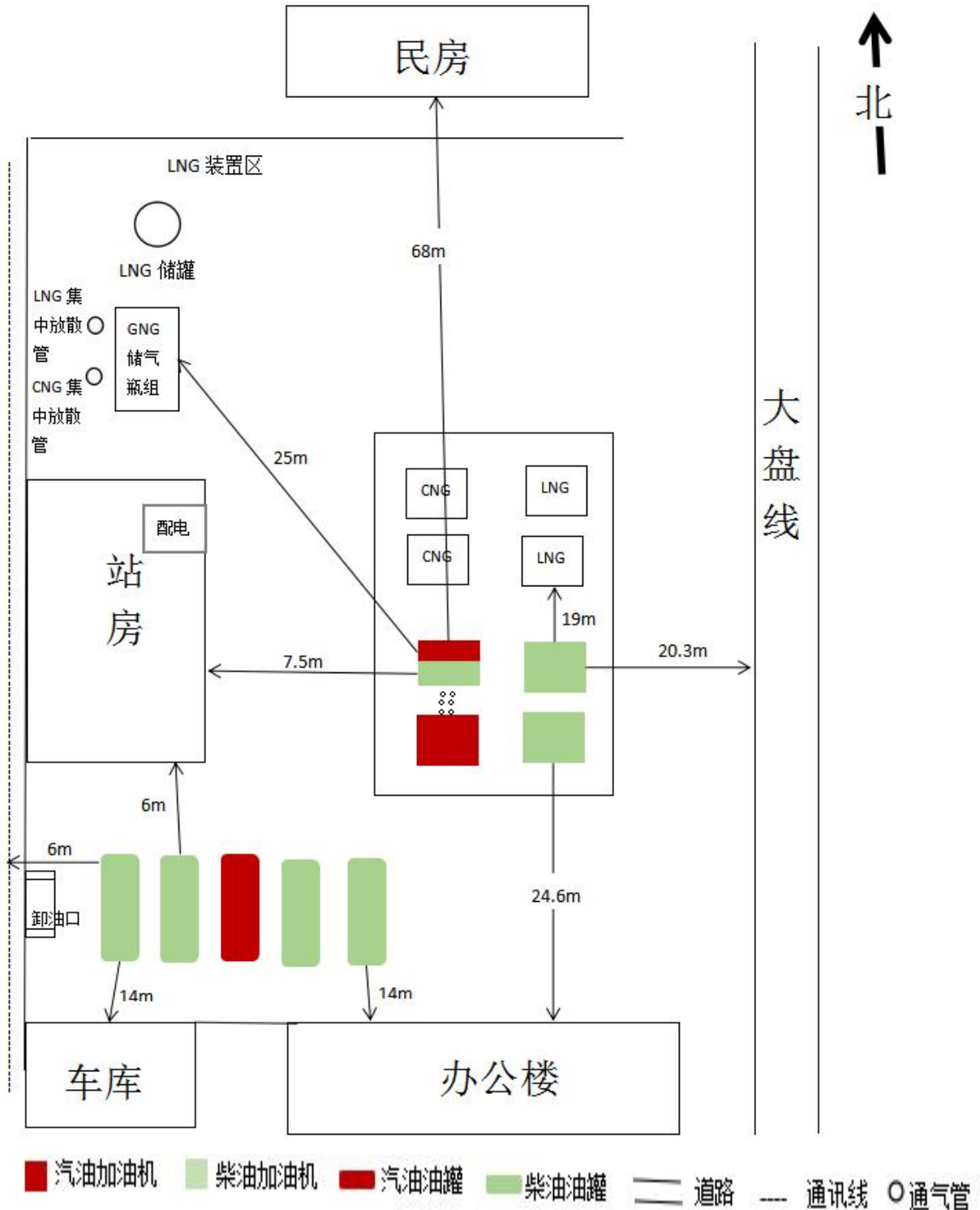
图 2.7.2-1 平面布置图
