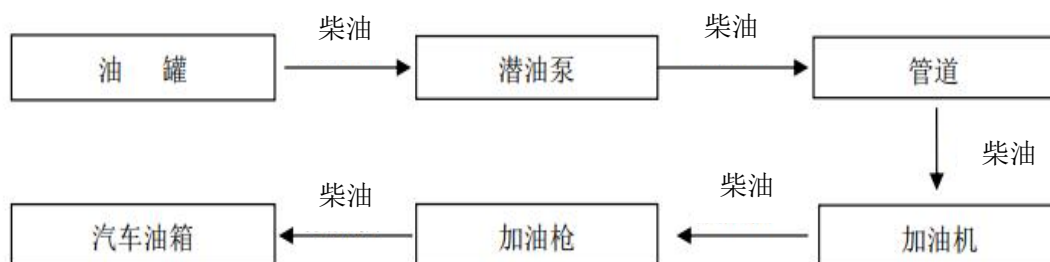
图 2.4.1-4 柴油加油工艺流程图
