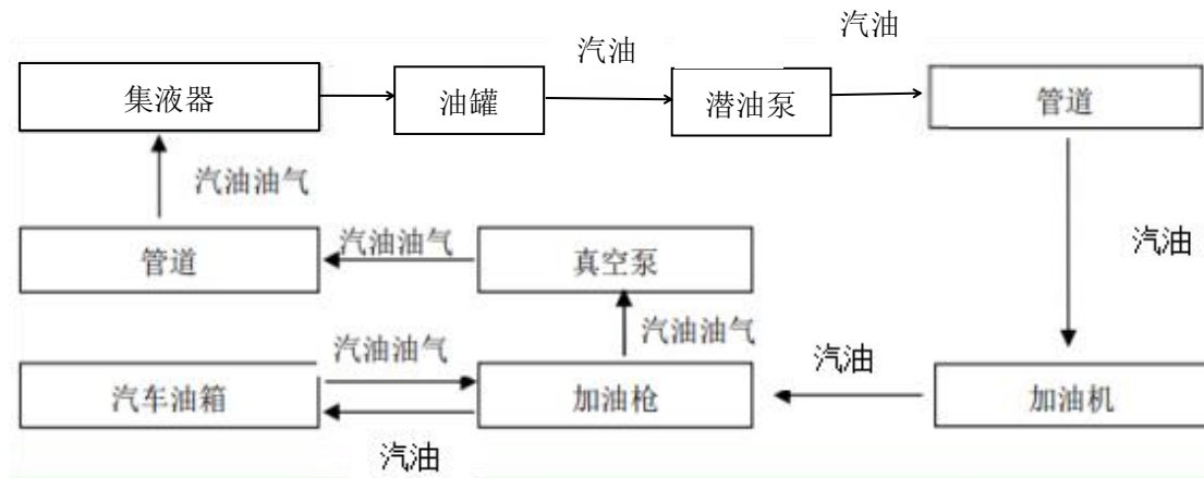
图 2.4.1-3 乙醇汽油加油及油气回收工艺流程图
