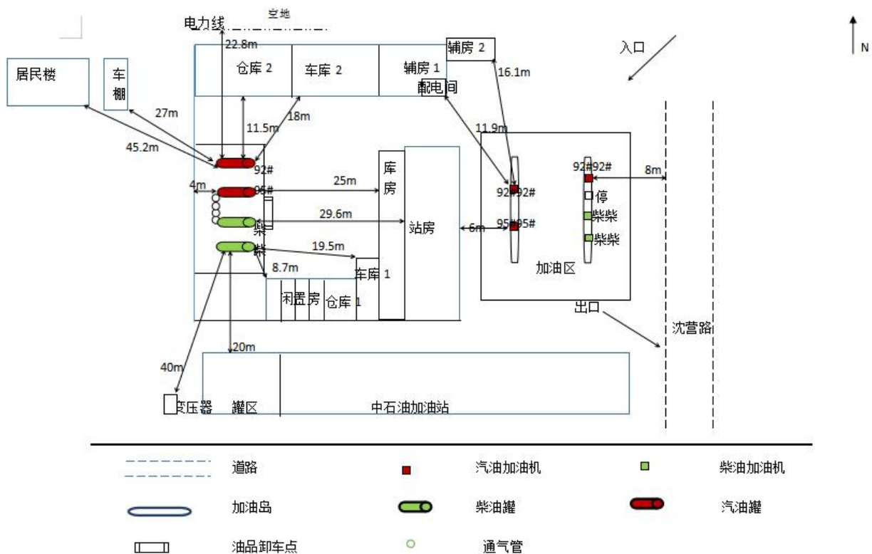
灯塔市春淼加油站 平面布置示意图
