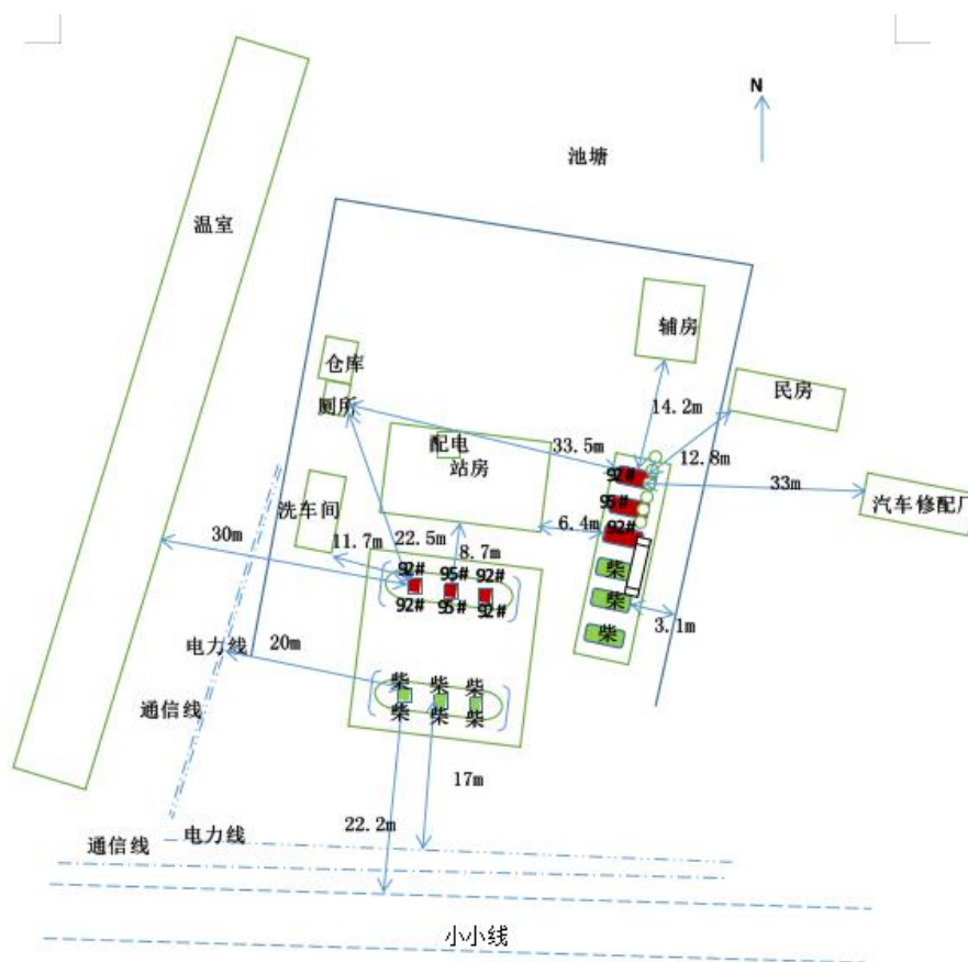
灯塔市经济开发区加油站平面示意图
