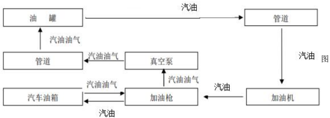
2.4.1-3 乙醇汽油加油及油气回收工艺流程图
