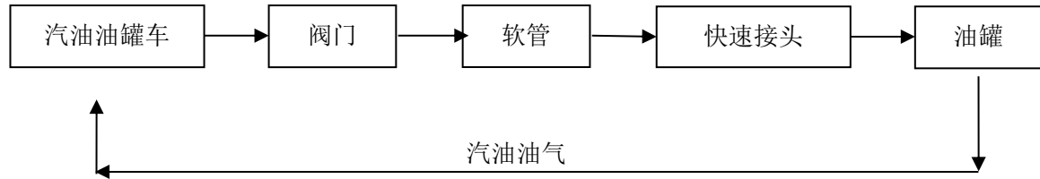
图 2.4.1-1 乙醇汽油罐车密闭卸油及卸油油气回收工艺流程图
