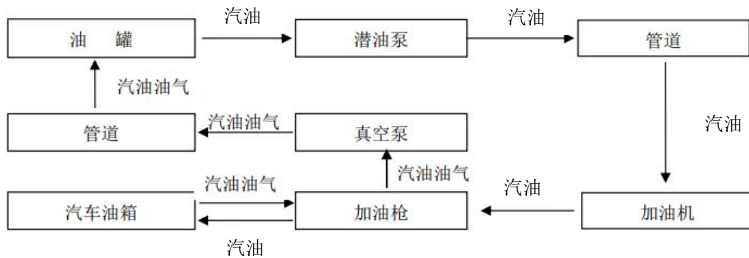
图 2.4.1-3 乙醇汽油加油及油气回收工艺流程图
