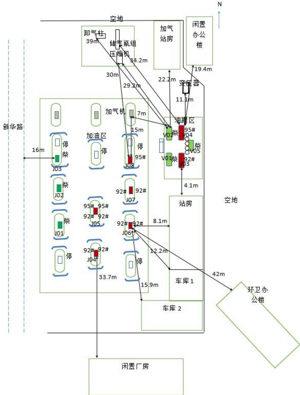
辽阳市太子河石油销售有限公司新华加油站平面示意图
