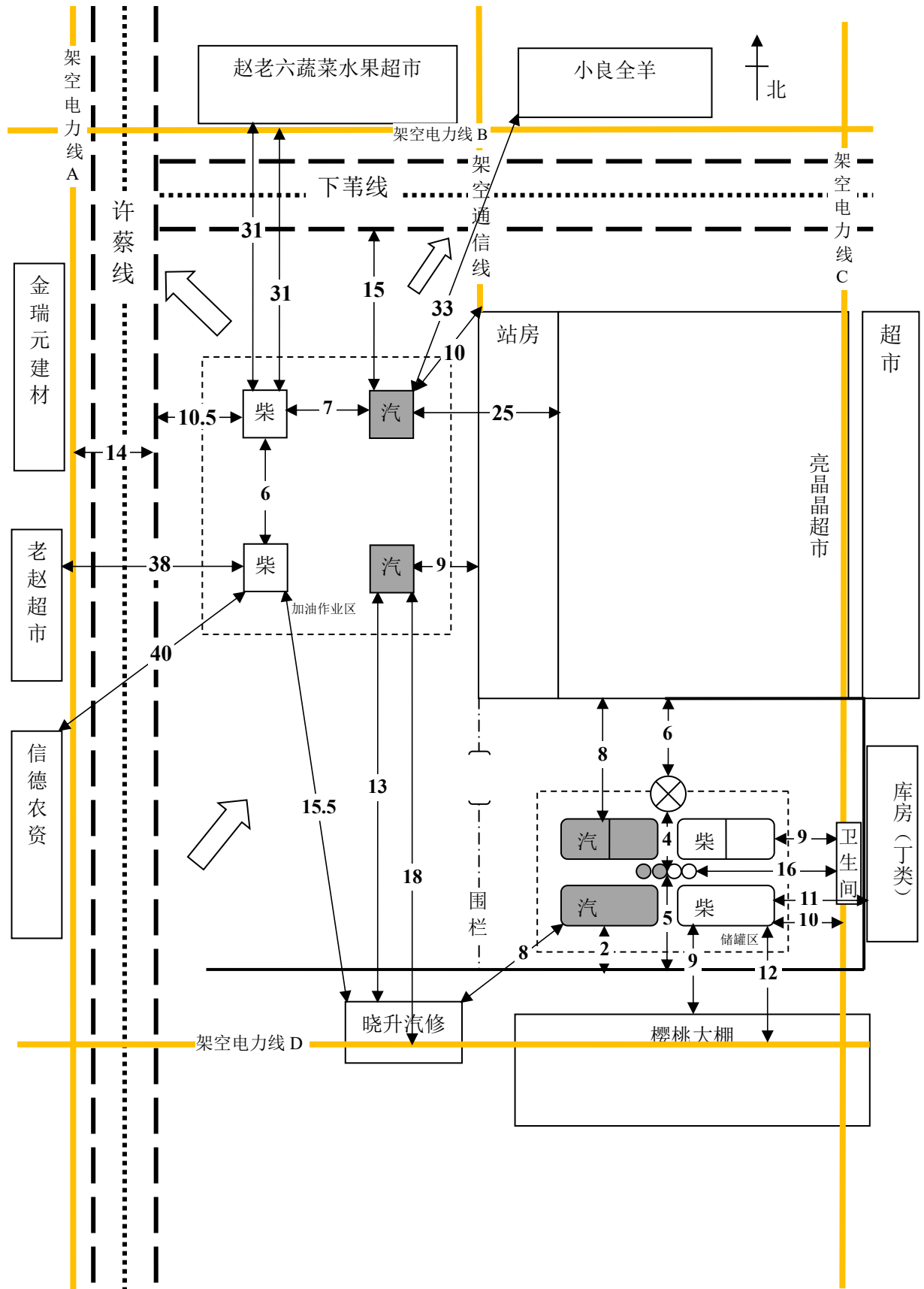
图 2.7.2-1 平面布置图
